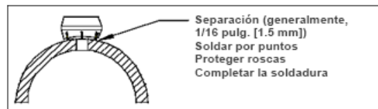
Figura 3. Separación para soldar
